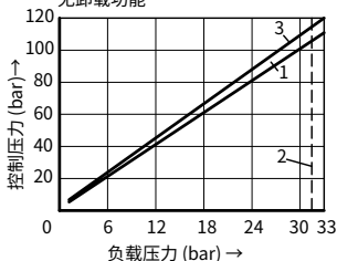
控制压力-负载压力曲线
